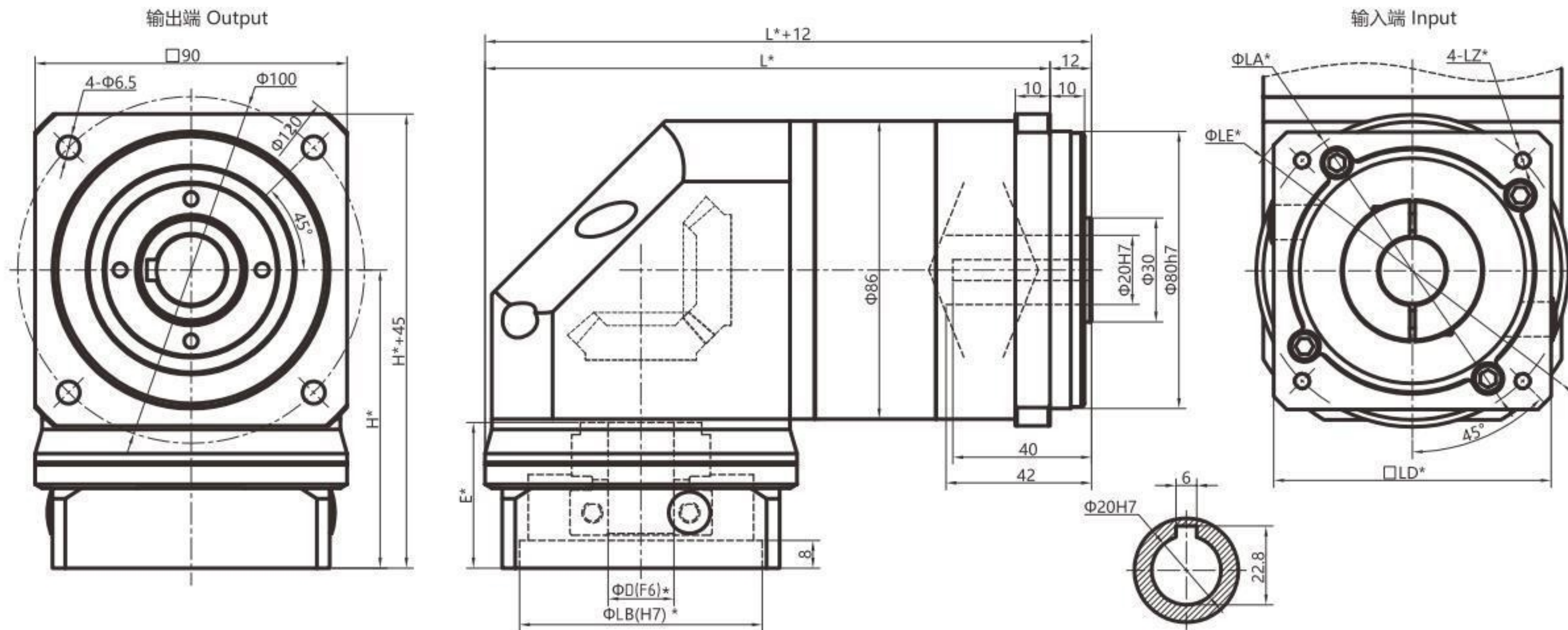
适配电机
